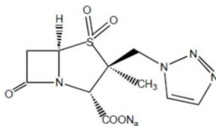
Tazobactam sodium
